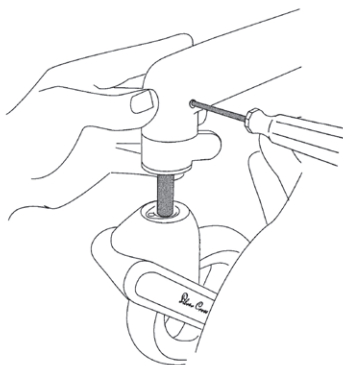
2. 本体を少し浮かせると取り外せます
